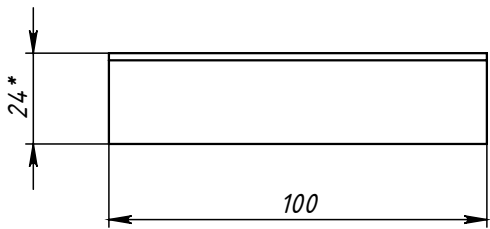
Поз.3 (Ложемент)
